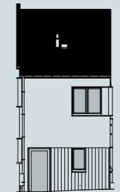
Pignon gauche
