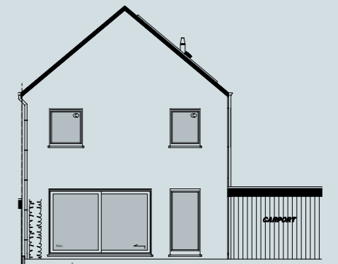
Pignon gauche
