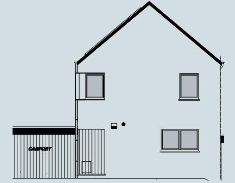
Façade avant
